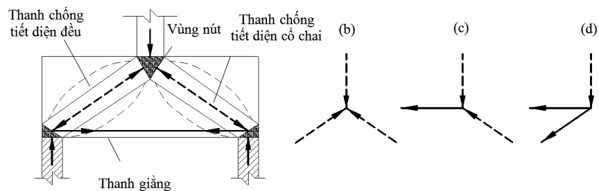
(b), (c), (d) Các kiểu nút trong mô hình giàn ảo (1-2)
