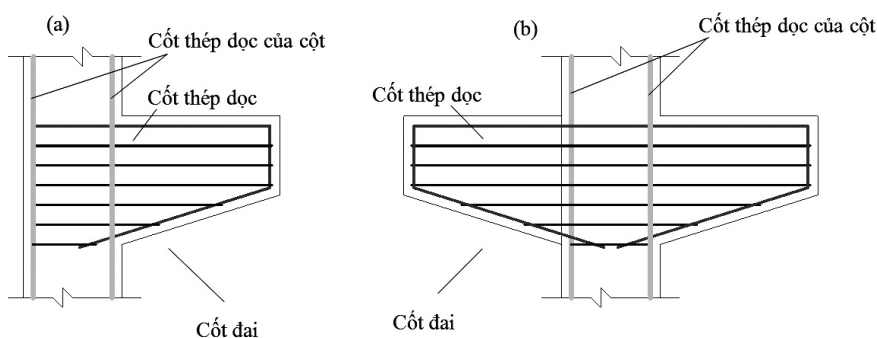
Hình 1: (a) Sơ đồ hình học vai cột đơn, (b) Sơ đồ hình học vai cột kép
