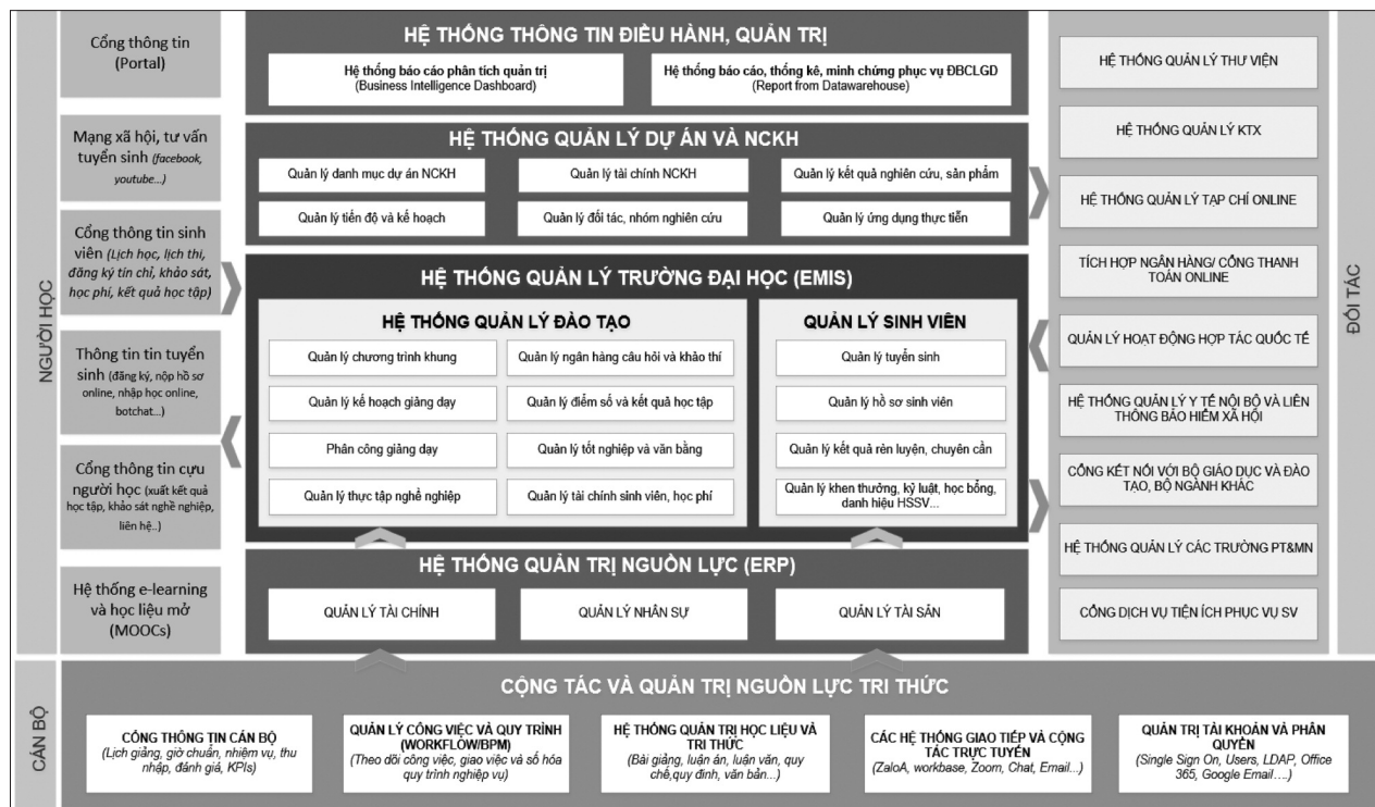
Hình 7: Kiến trúc ứng dụng của HNUE
