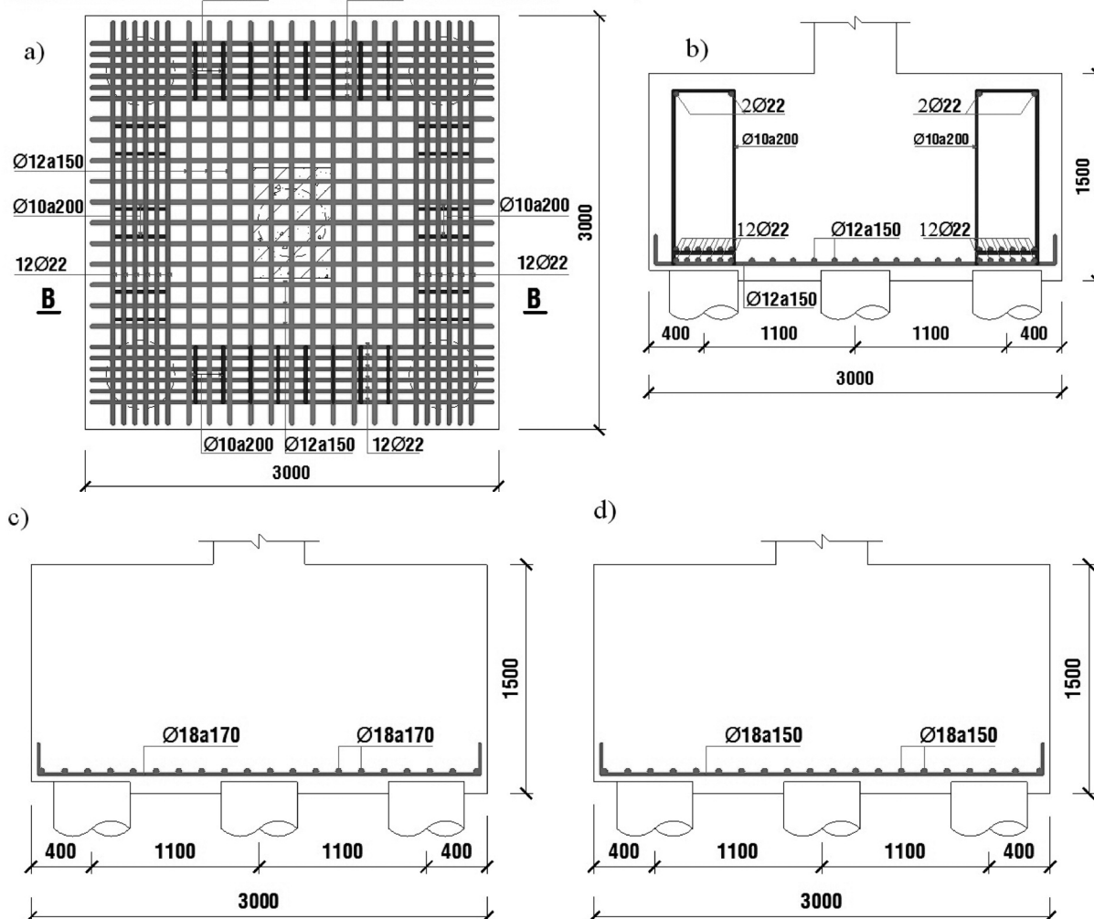
Hình 6: Bố trí cốt thép đài móng cọc. a), b) Theo STM 3D; c) Theo STM 2D; d) Theo mô hình dầm công xôn
