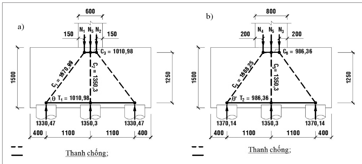
Hình 3. a), b) Mô hình giàn ảo phẳng đài móng cọc theo phương x và phương y (tác giả thực hiện, 2021)
