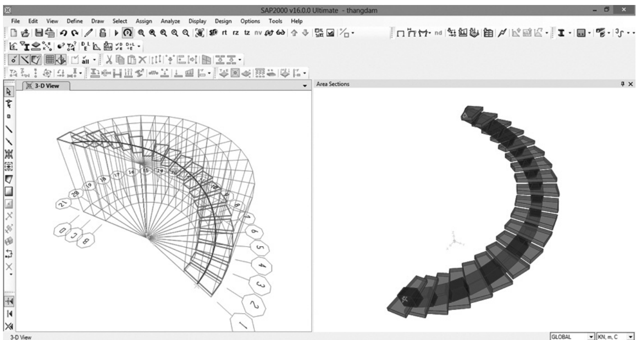
Hình 19: Kết quả mô hình cầu thang dạng dầm chịu lực (dạng xương cá)
