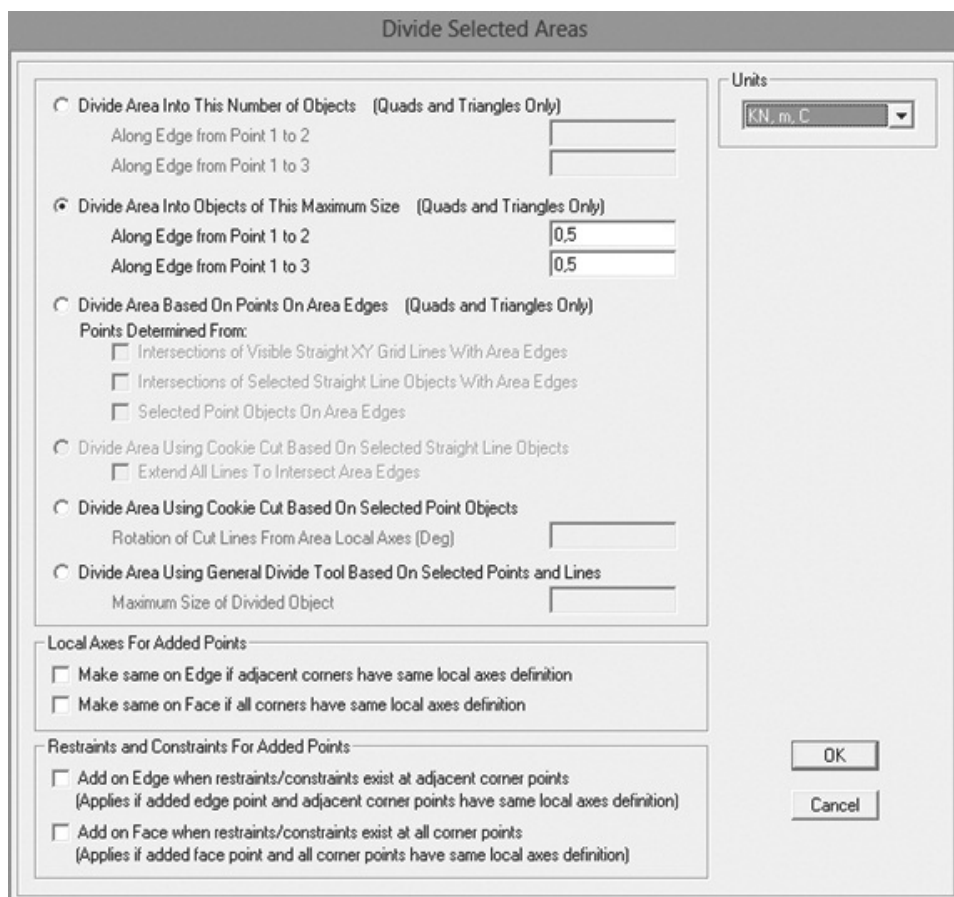
Hình 8: Hộp thoại Divide Selected Areas
