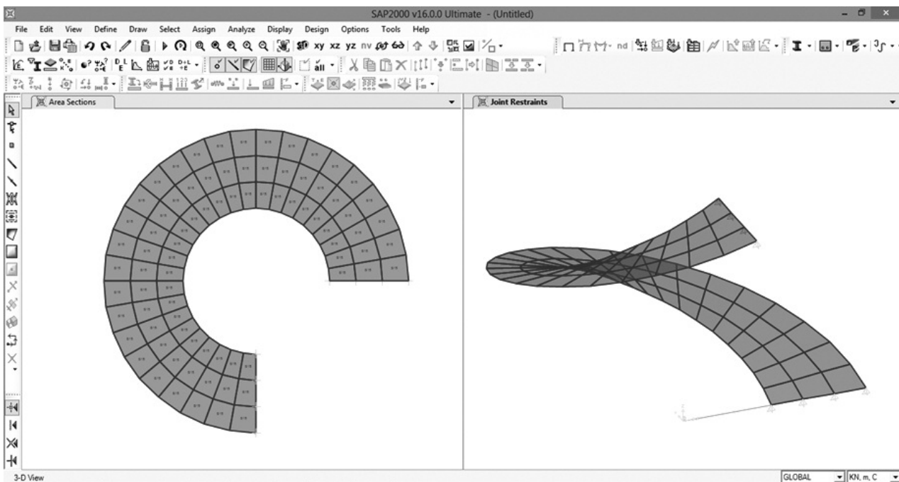
Hình 10: Kết quả mô hình
