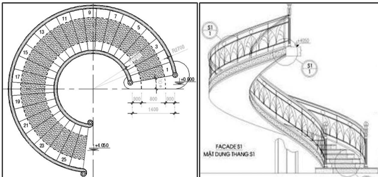
Hình 2: Mặt bằng và hình dạng cầu thang lượn dạng bán nguyệt chịu lực
