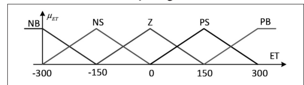
Hình 3: Hàm liên thuộc ngồ vào ET
