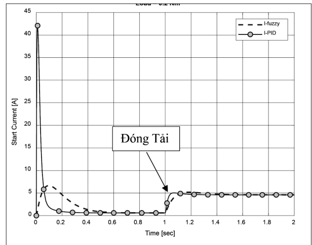
Hình 9: Đáp ứng dòng điện có tải của bộ điều khiển PID và Thông minh
