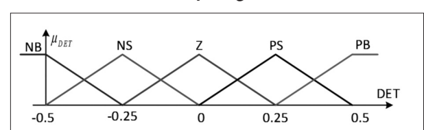
Hình 4: Hàm liên thuộc ngồ vào DET
