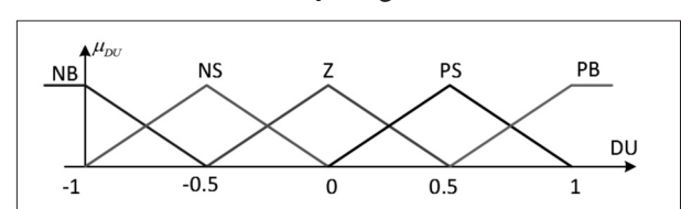
Hình 5: Hàm liên thuộc ngồ ra Du
