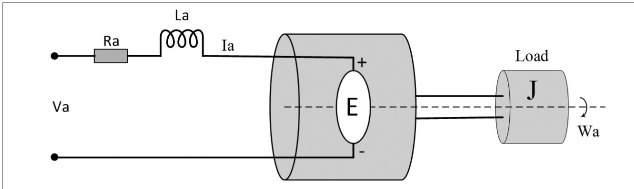
Hình 1: Mô hình động cơ DC kích từ độc lập
